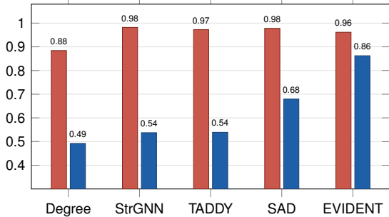
Bitcoin-OTC
