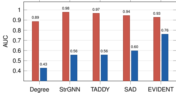
Bitcoin-Alpha
