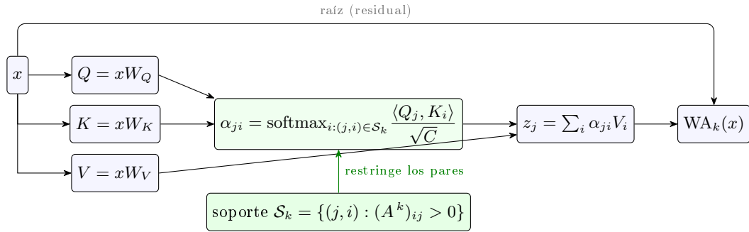
Figura 2. Una capa de Walk Attention a alcance k . Consultas, claves y valores son mapas lineales de los atributos; la atención se calcula solo sobre los pares alcanzables \mathcal{S}_k que provee el álgebra de caminos (el patrón de no-ceros de A^k ), se agrega y se suma un término raíz residual. La caja verde del soporte distingue a Walk Attention de la atención densa (todos los pares) y de la de un salto (aristas).
