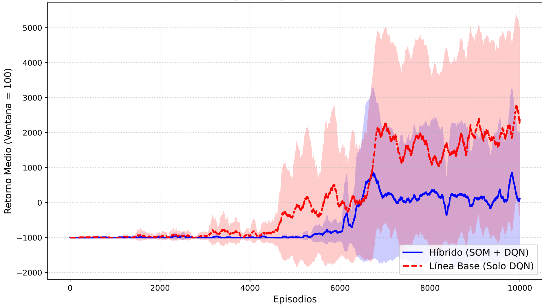
Curva de Aprendizaje: Híbrido vs Línea Base
