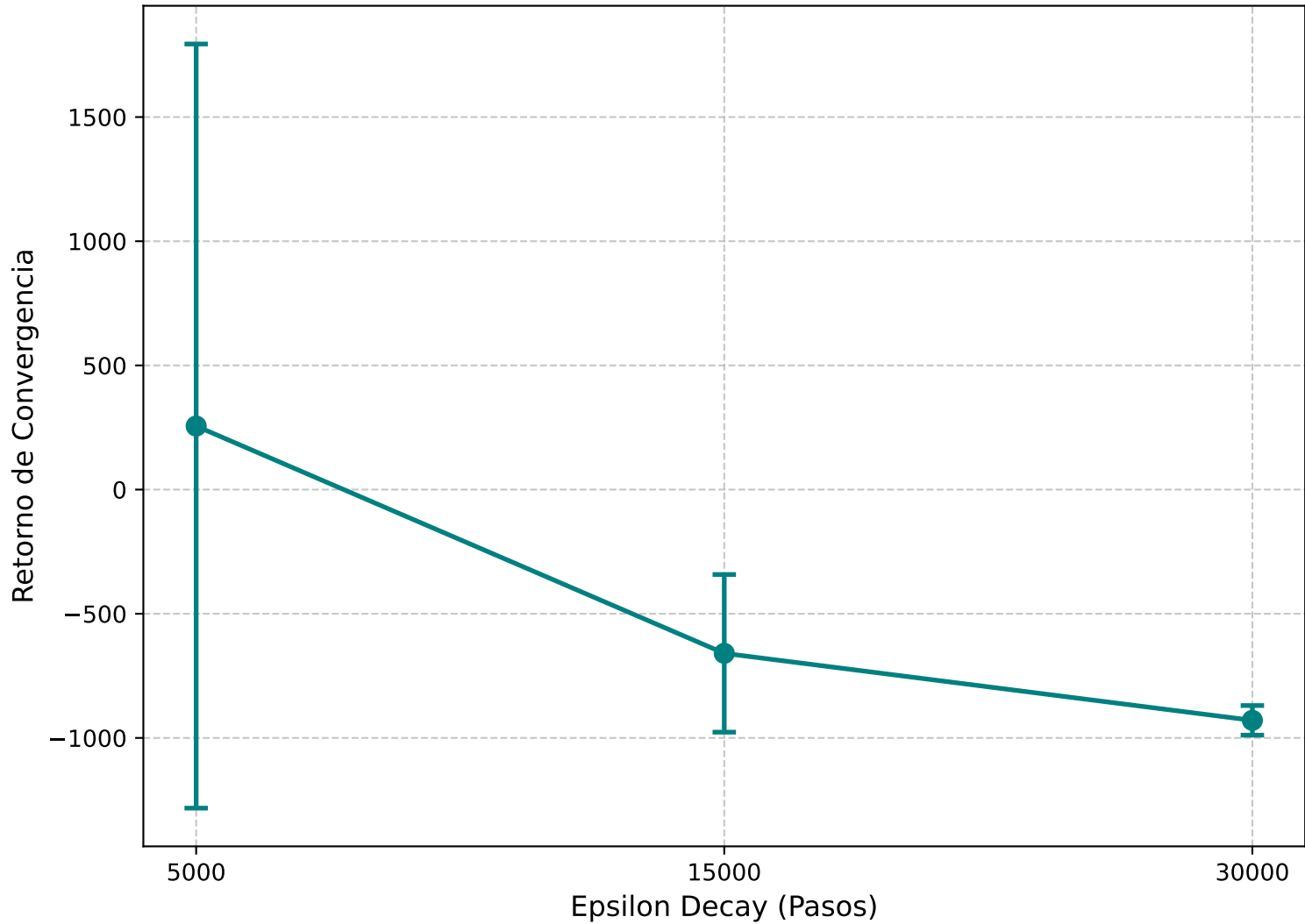
Efecto del Decaimiento de Epsilon (DQN)
