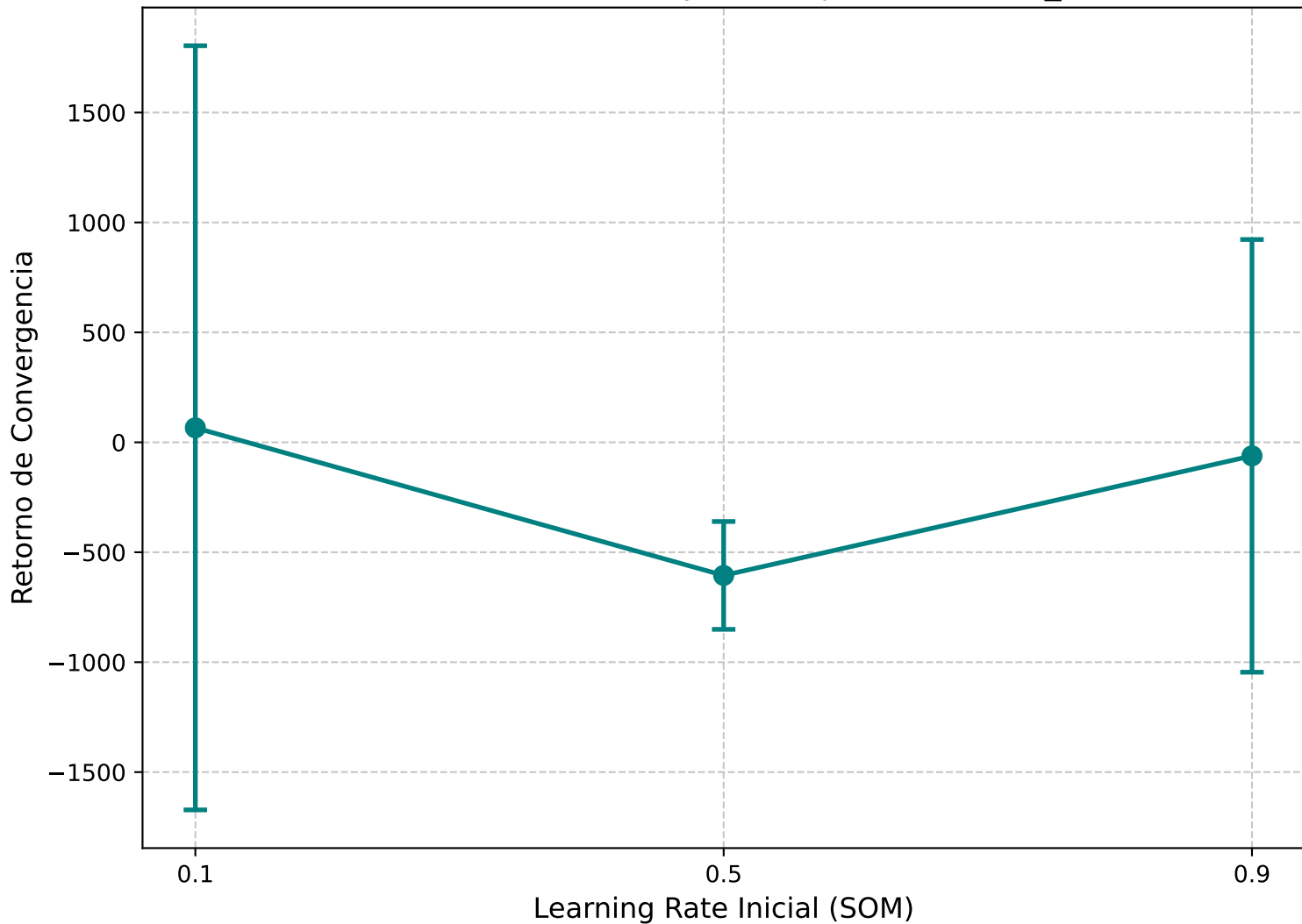
Efecto de la Tasa de Aprendizaje del SOM (lr_init)
