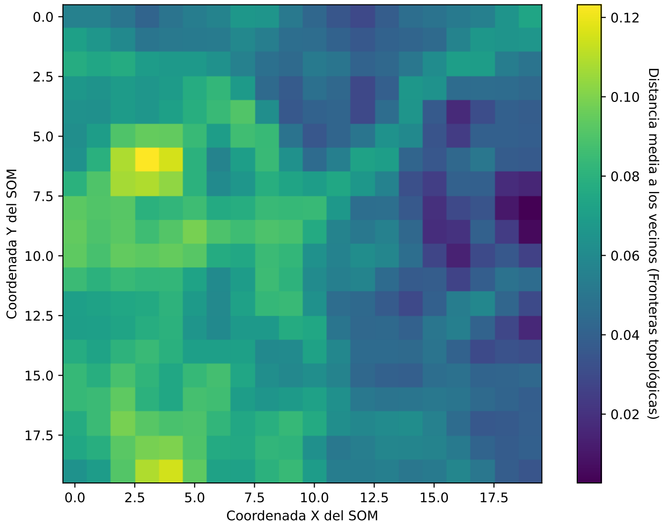
Dinámica Interna (U-Matrix) - SOM 20x20 (Semilla 1)
