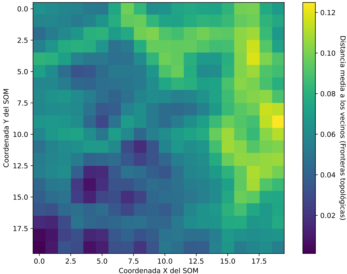
Dinámica Interna (U-Matrix) - SOM 20x20 (Semilla 42)
