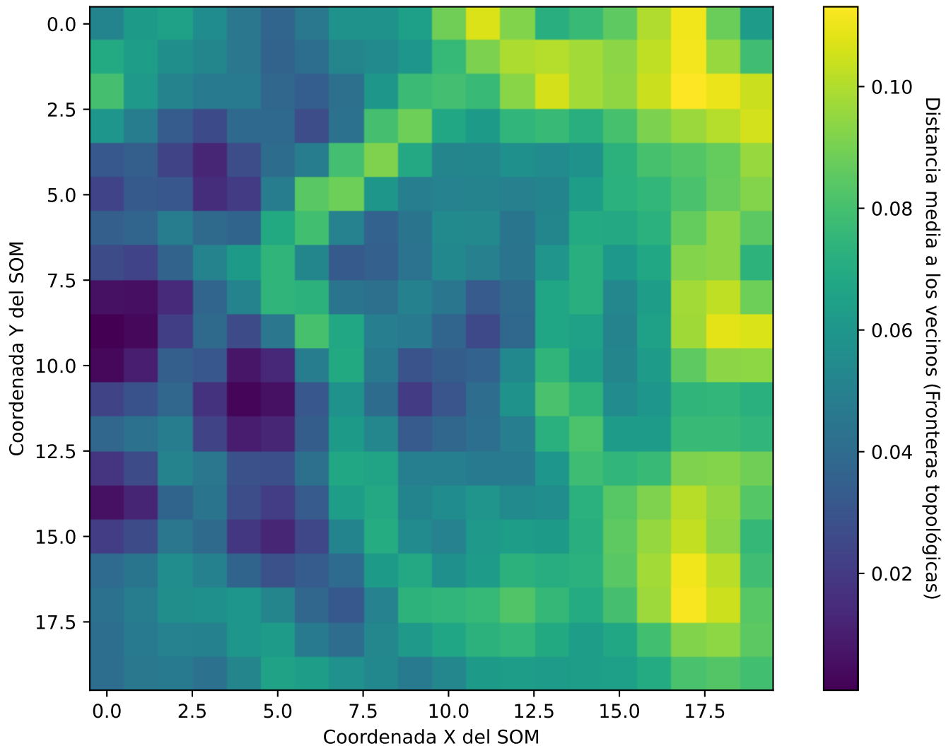
Dinámica Interna (U-Matrix) - SOM 20x20 (Semilla 7)
