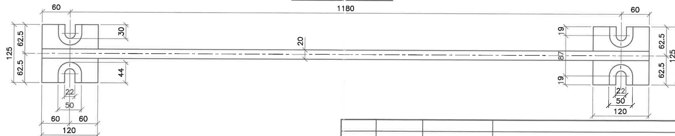
- Coupe BB -
