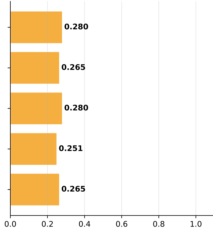
F1@10
