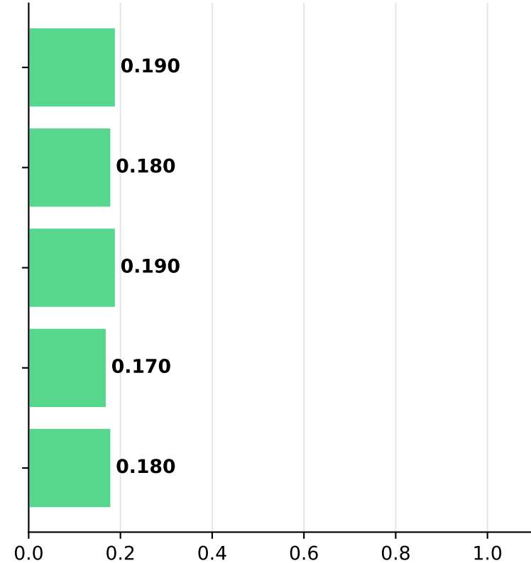
P@10
