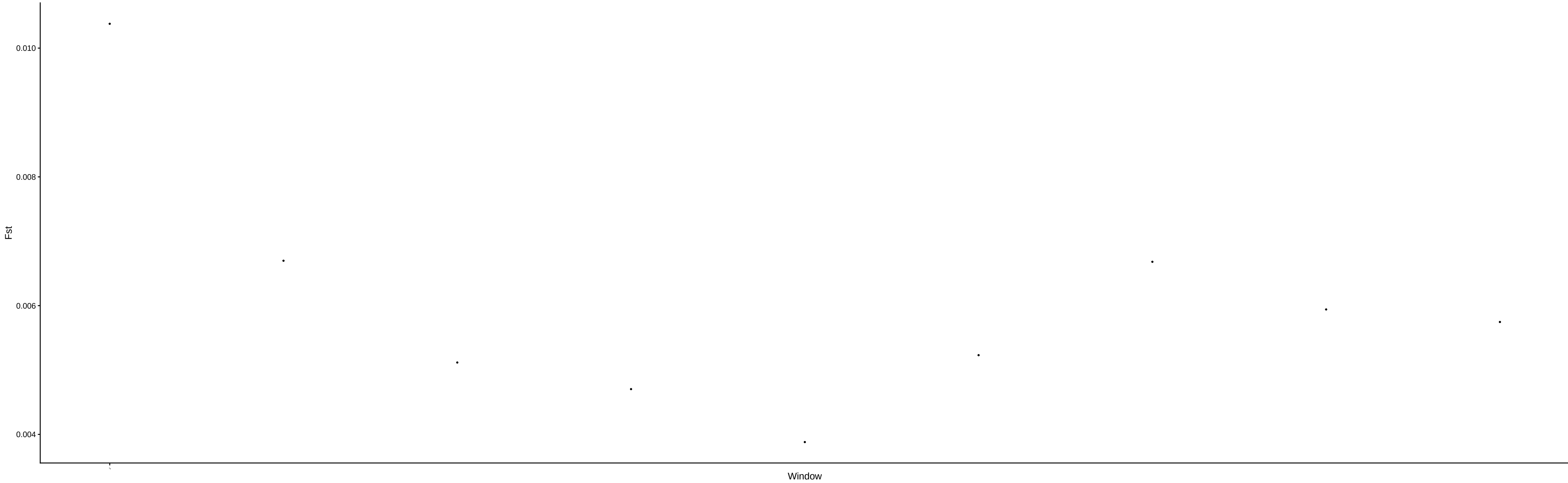
FST for Scaffold: JAKZJL020000158.1
