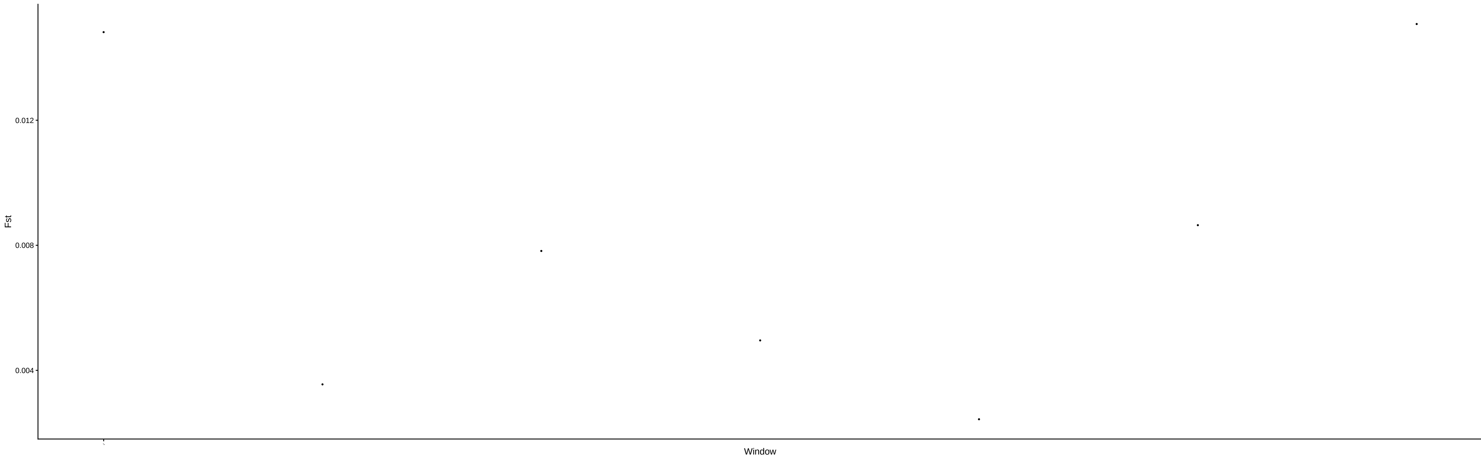
FST for Scaffold: JAKZJL020000174.1
