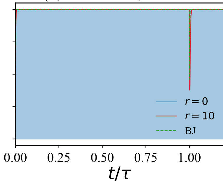
(d) trotterized, r = 10
