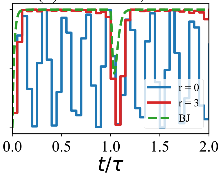
(d) trotterized, r = 3
