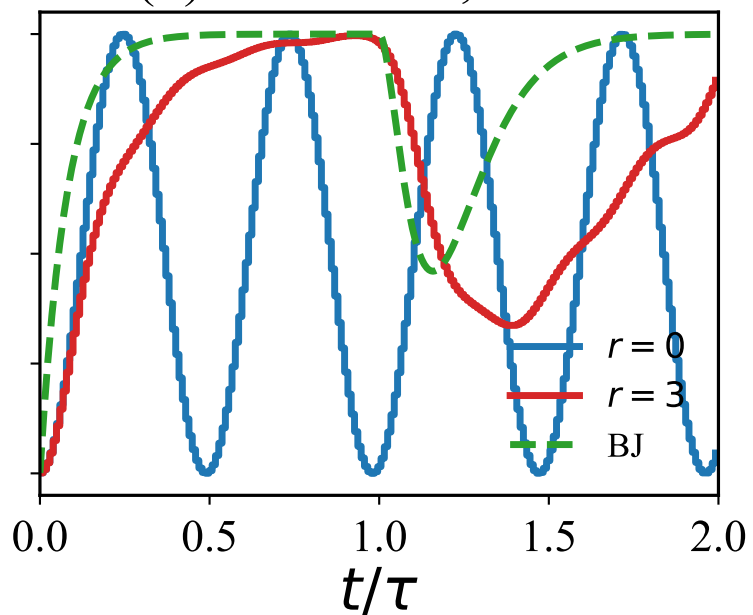
(d) trotterized, r = 3
