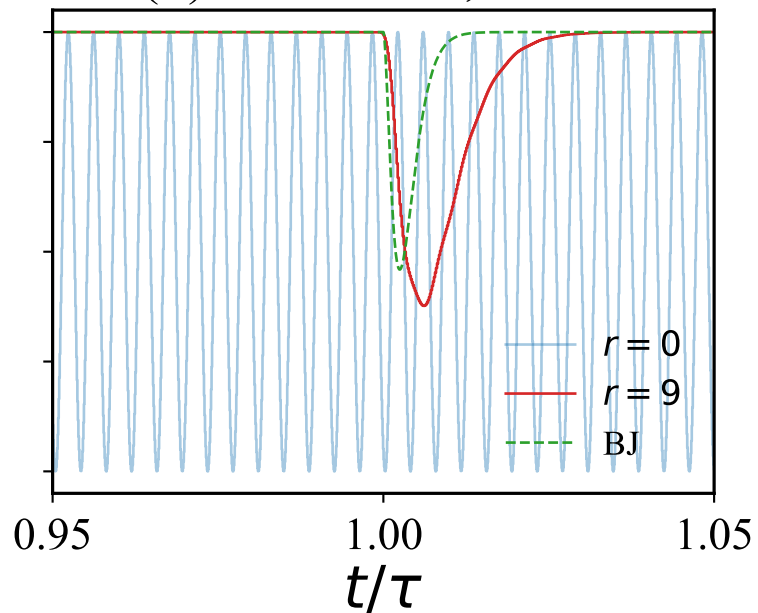
(d) trotterized, r = 9
