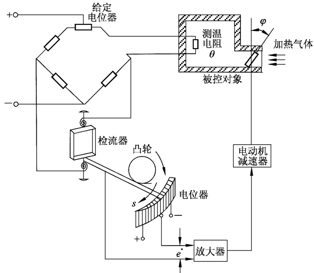
炉温采样控制系统原理图
