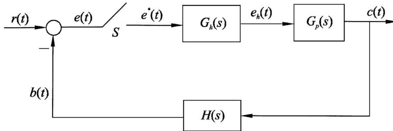
采样系统典型结构图
