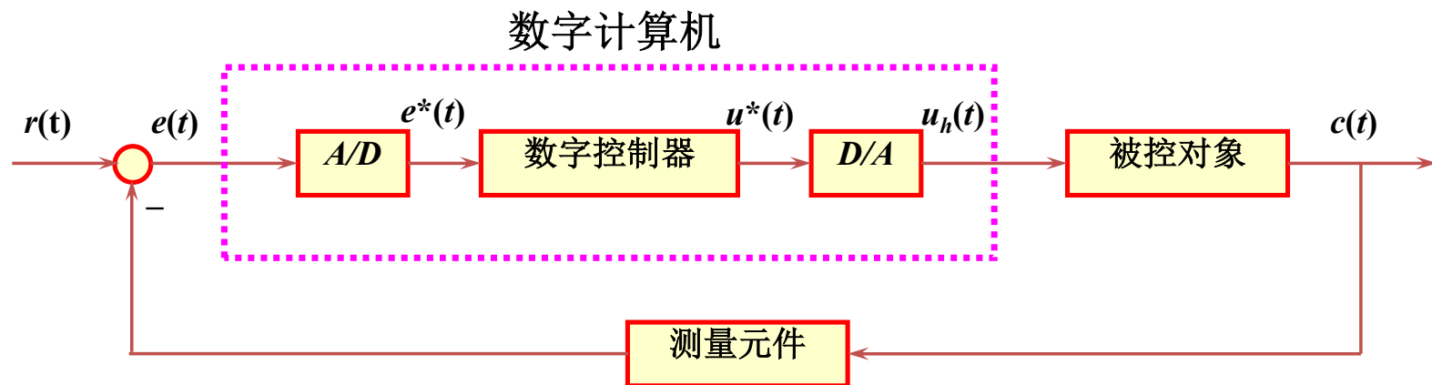
计算机控制系统典型原理图
