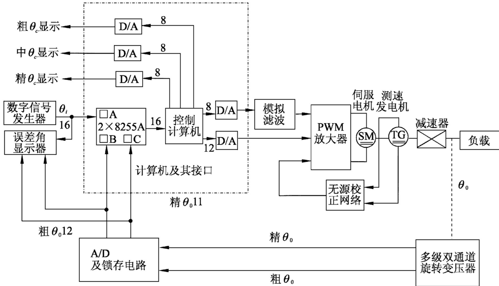
小口径高炮高精度伺服系统
