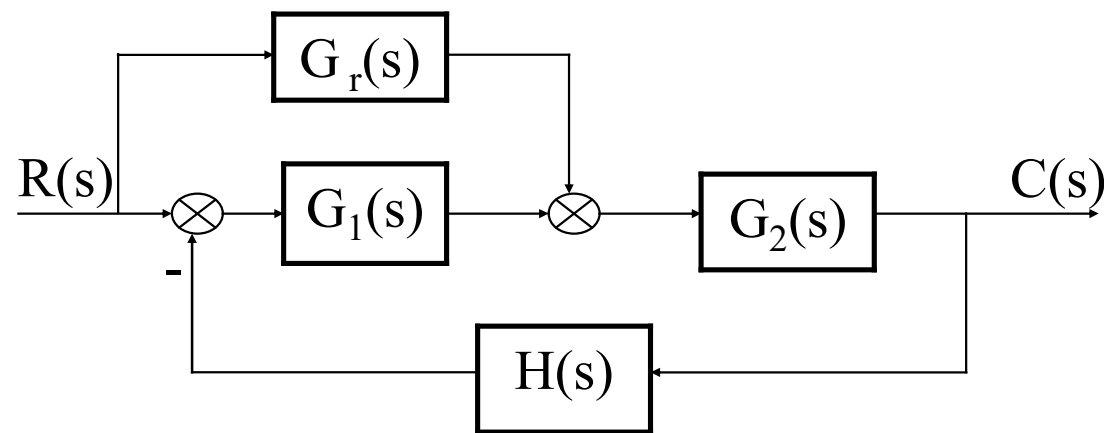
按输入补偿的复合控制
