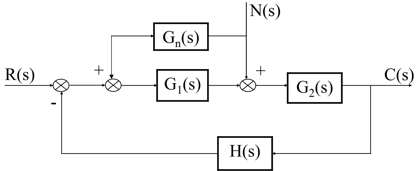
按扰动补偿的复合控制
