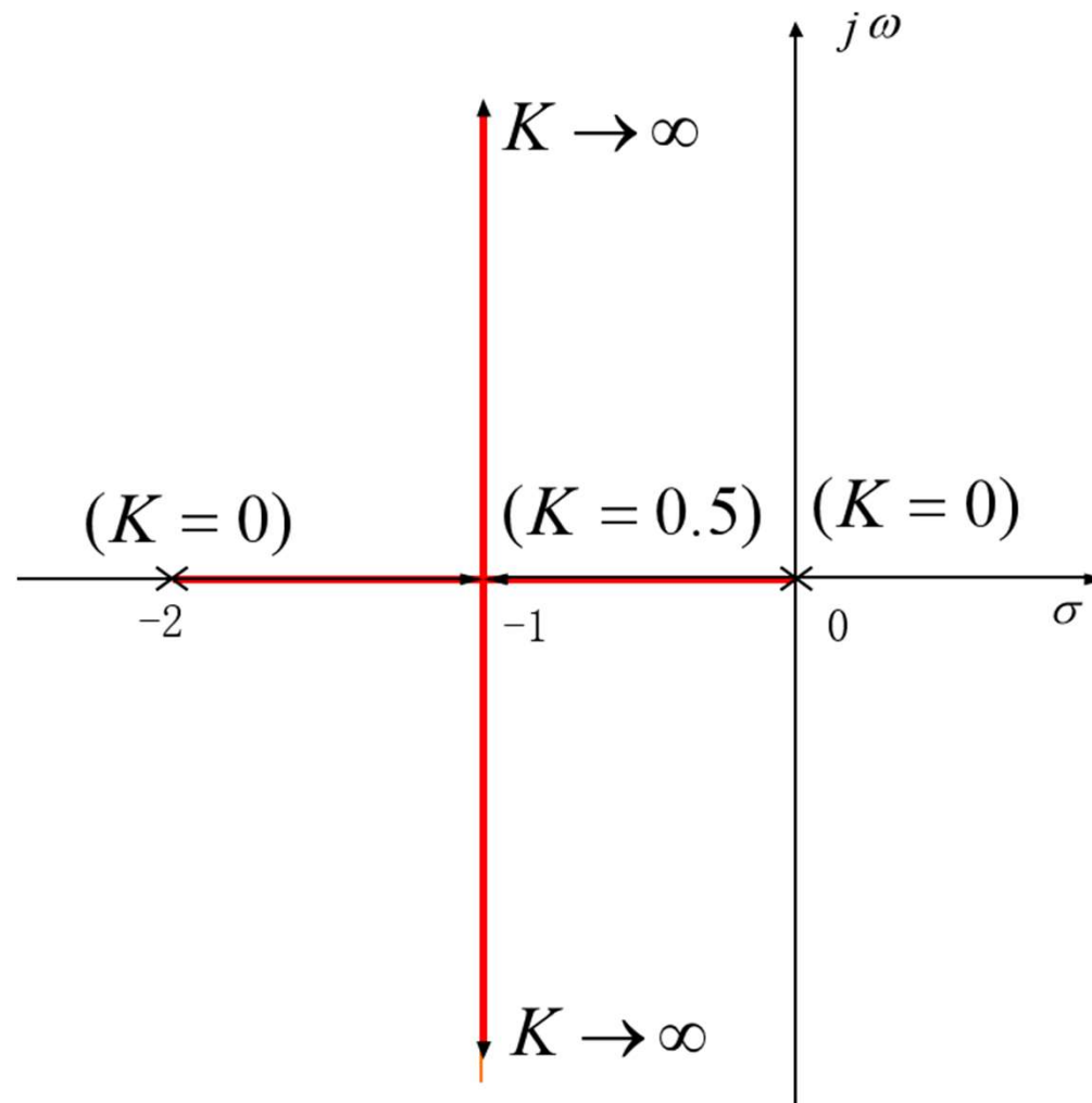
系统的根轨迹
