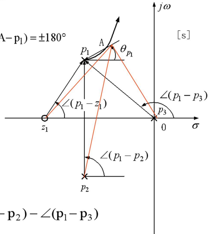
图 起始角 \theta_{p_1} 的求取
