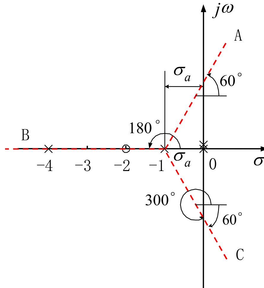
图 根轨迹的渐近线
