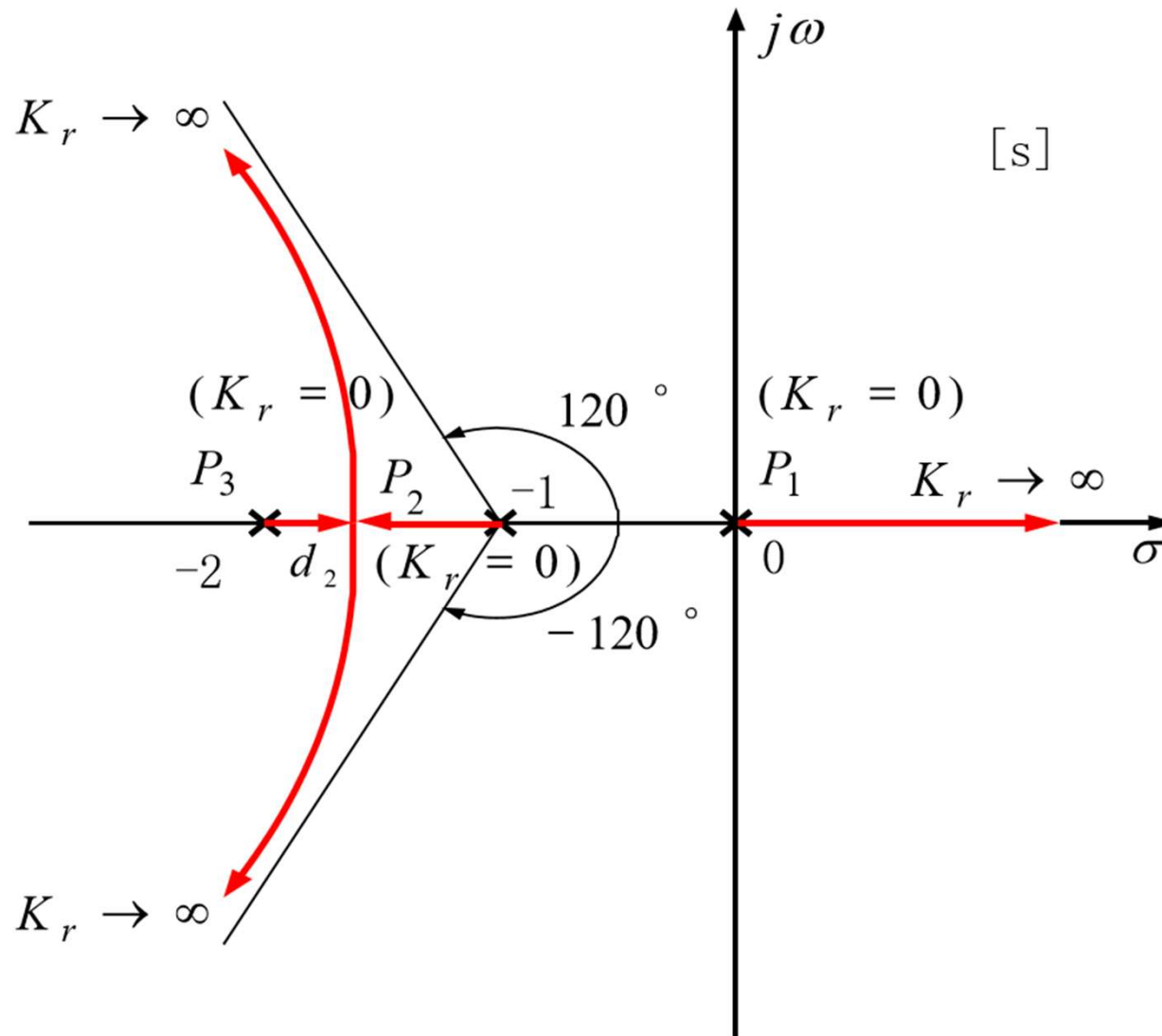
图 正反馈系统的根轨迹
