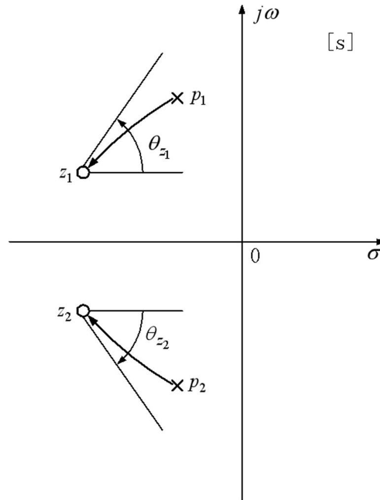
图. 根轨迹的终止角
