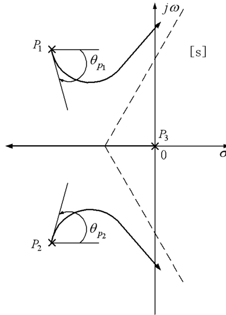
图. 根轨迹的起始角
