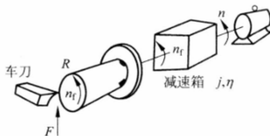
图 2.15 车床切削示意图
