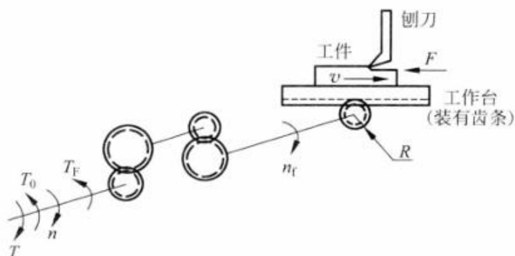
图 2.4 刨床电力拖动示意图
