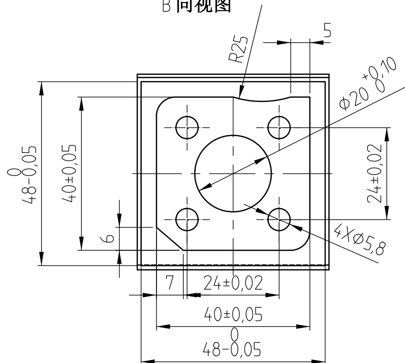
B 向视图
