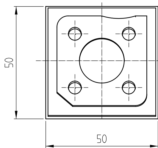
B 向视图
