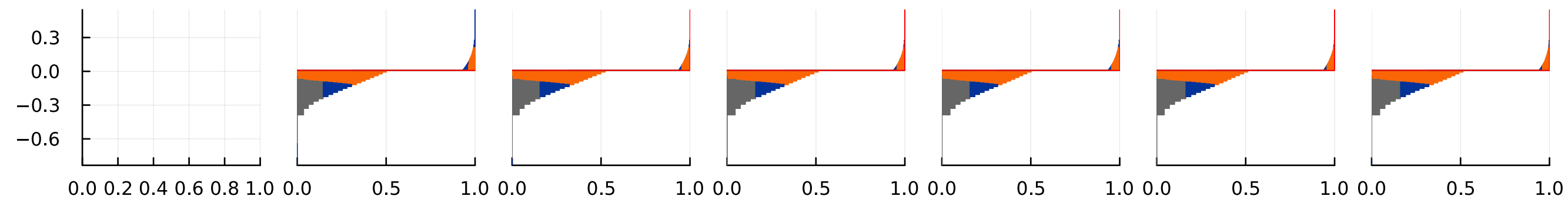
SSP 1.26
