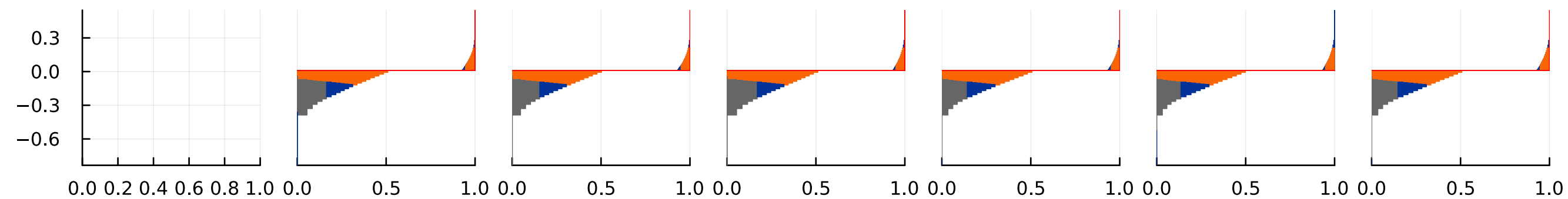
2021 - 2031
