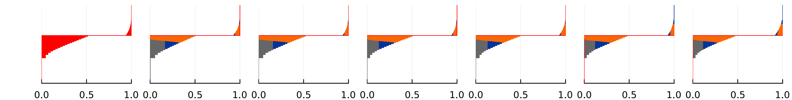
SSP 3.70
