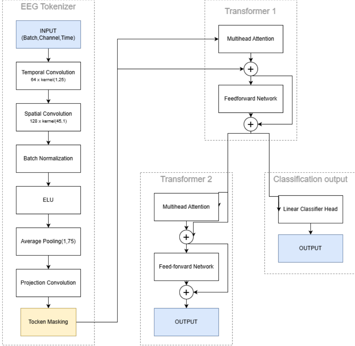
Figura 3.2: Esquema de la arquitectura de MiRepNet para entrenamiento.
