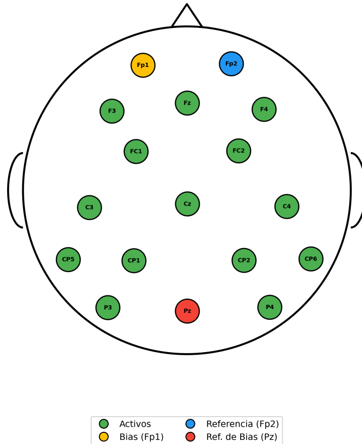
Figura 4.1: Disposición de electrodos del casco BrainAccess HALO.
