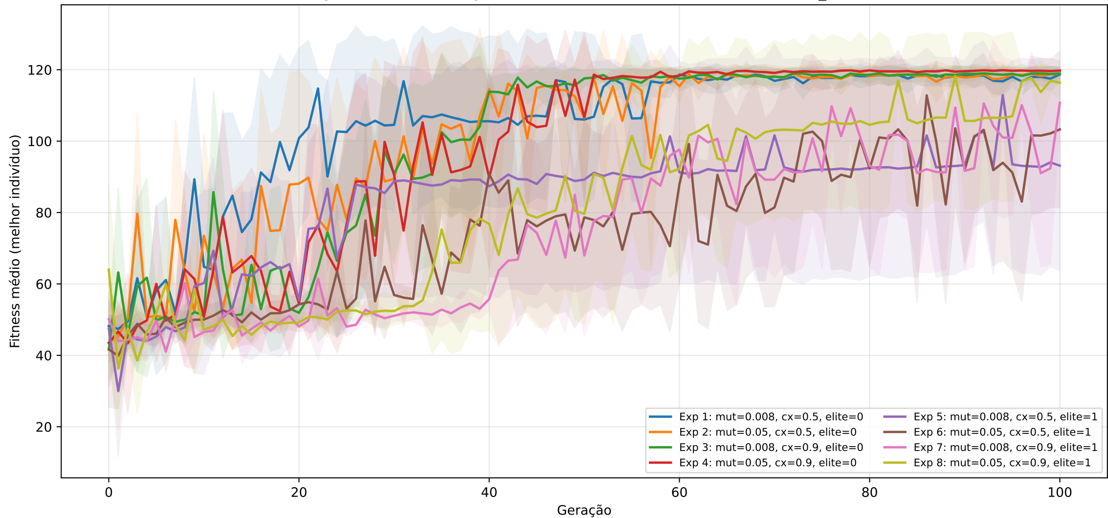
Comparação das 8 Experiências — Fitness Médio ( \pm 1\sigma ) [sem_vento]
