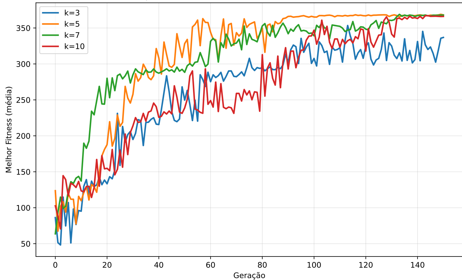
Impacto do Tamanho do Torneio (média de 3 runs)
