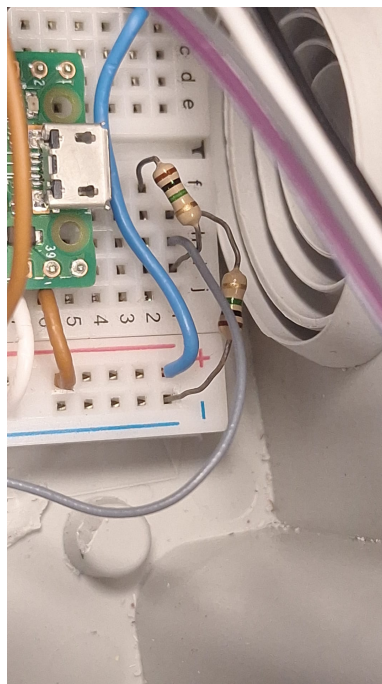
Figura 4: Fotografia do circuito do divisor de tensão.
