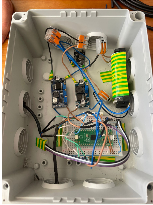
Figura 5: Fotografia do interior da caixa, já com todos os componentes montados.
