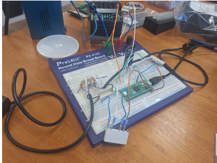
Figura 1: Fotografia do circuito montado em placa de desenvolvimento (Protótipo 0).
