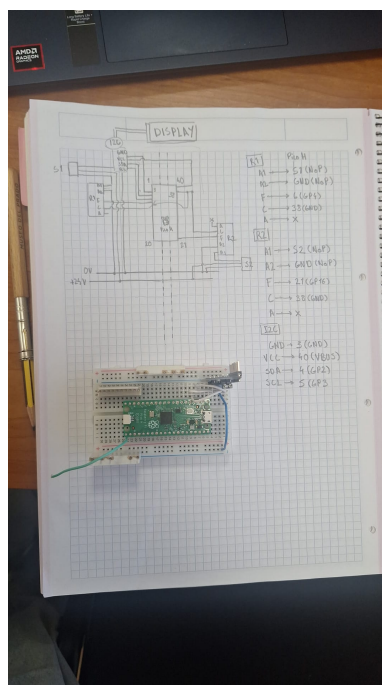
Figura 9: Fotografia do Protótipo 0 junto ao caderno de anotações do desenvolvimento.
