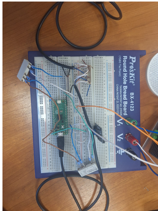
Figura 8: Fotografia do Protótipo 0 em placa de desenvolvimento (vista de cima).
