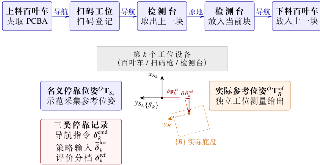
图 9: PCBA 上下料五子任务链与工位停靠误差的定义
