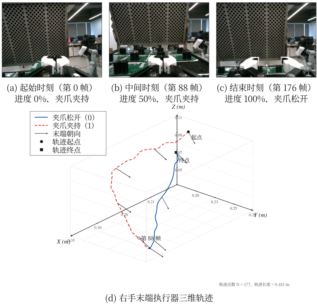
图 14: 将 PCBA 放置到百叶车任务的示例观测、右机械臂末端执行器轨迹与夹爪状态
