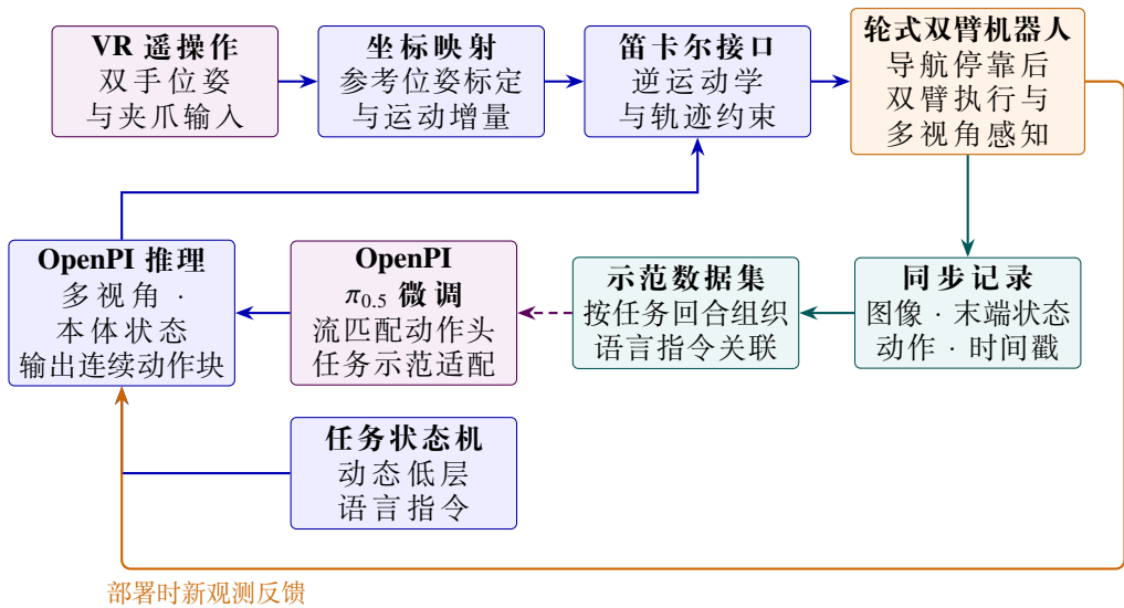
图 13: 已贯通的 VR 数采- \pi_{0.5} 微调-OpenPI 推理-真机执行接口链路
