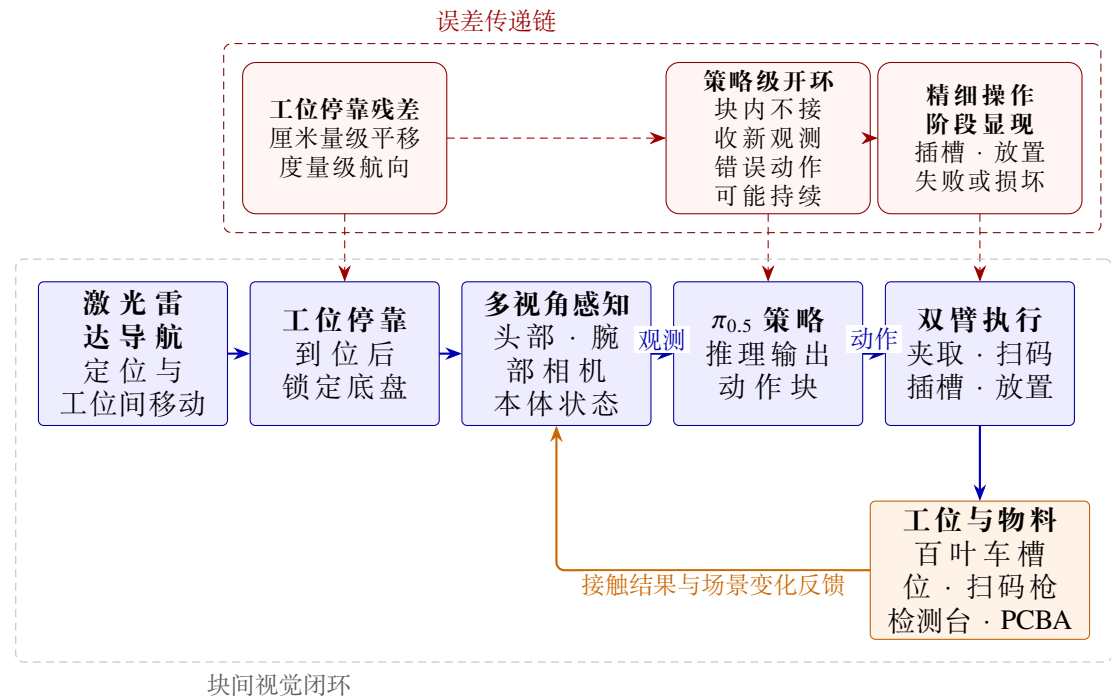
图 4: PCBA 上下料任务中的模仿学习策略闭环与工位停靠残差传递链
