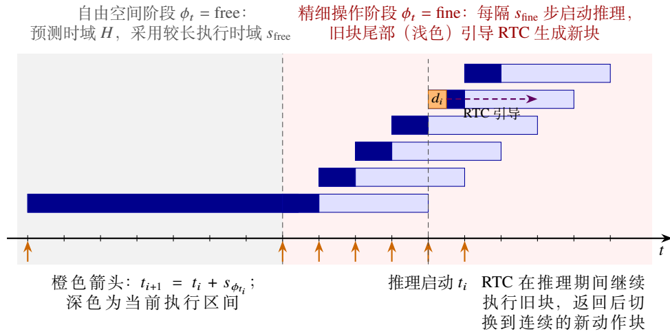
图 10: 分阶段执行时域与 RTC 跨动作块连续衔接时序
