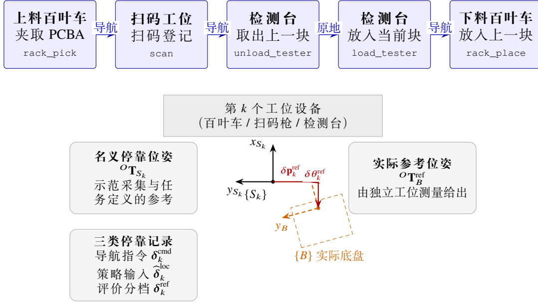
图 9: PCBA 上下料五子任务链与工位停靠残差的定义
