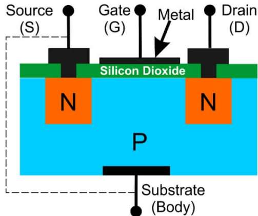
Figure: Diagrama de sección transversal de un FET
