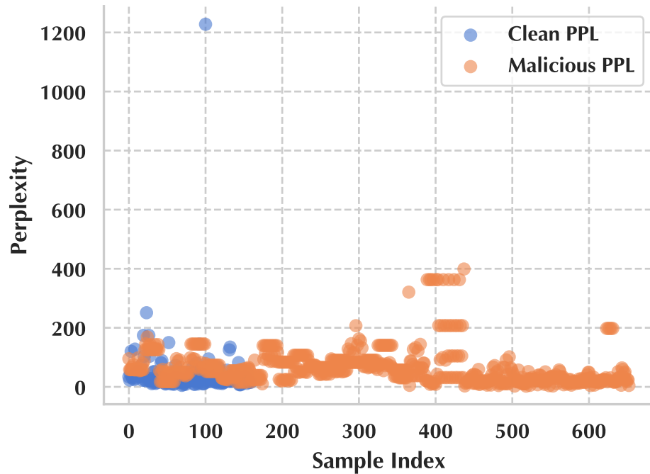
Llama 3.2-8B
