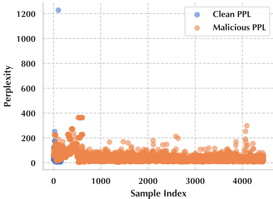
GPT-4o
