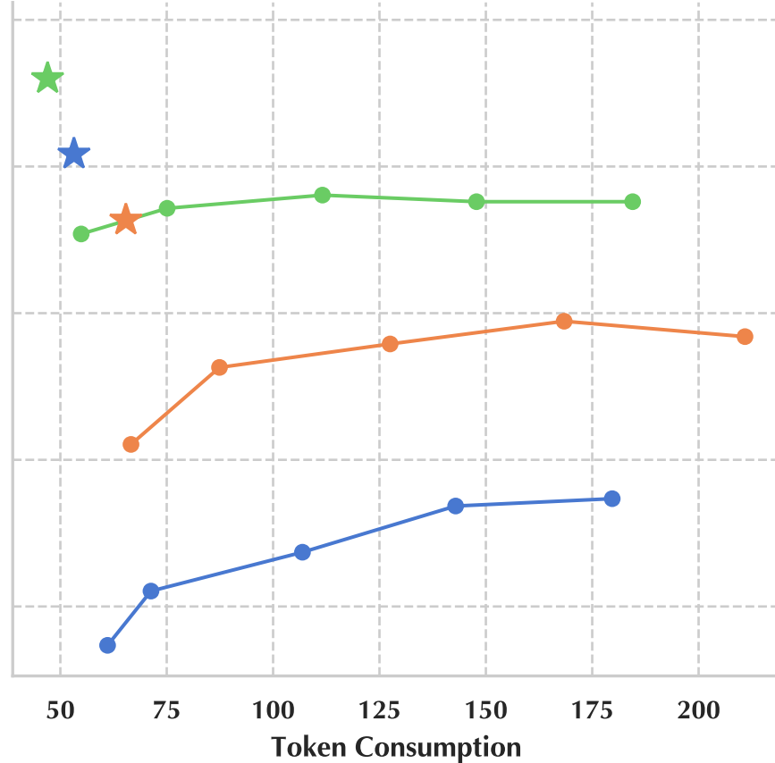
LLaMA 3.2-8B
