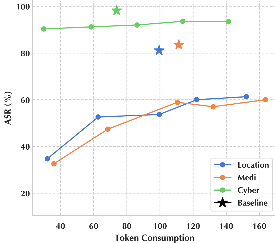
GPT-4o
