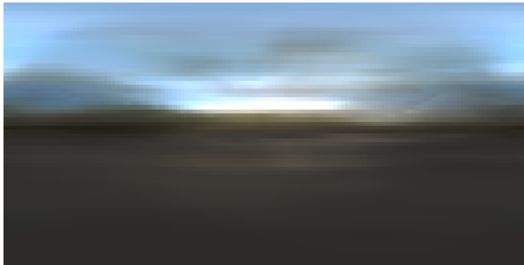
RENI++
