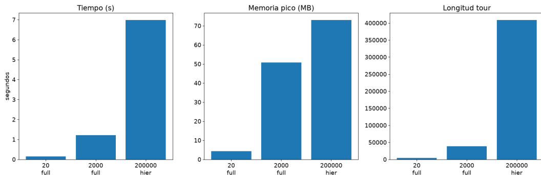
Figura 2: Tiempo, memoria pico y longitud del tour para los tres tamaños.
