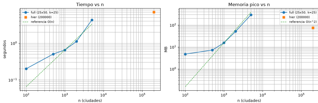
Figura 3: Tiempo y memoria frente a n (log-log) con referencias O(n) y O(n^2) , más el punto jerárquico de 200000.
