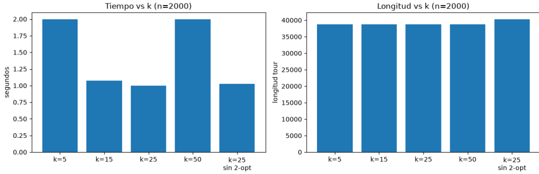
Figura 4: Tiempo y longitud según k ( n=2000 ), con variante sin 2-opt.
