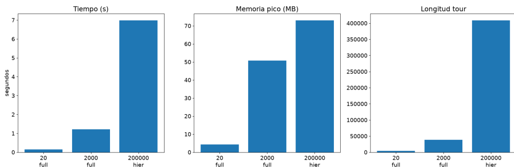
Figura 2: Tiempo, memoria pico y longitud del tour para los tres tamaños.
