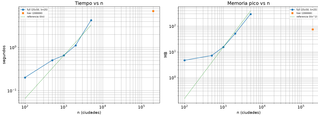
Figura 4: Tiempo y memoria frente a n (log-log) con referencias O(n) y O(n^2) , más el punto jerárquico de 200000.
