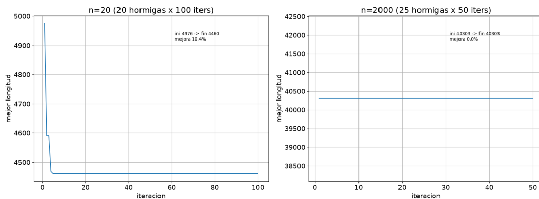
Figura 3: Mejor longitud global por iteración, n=20 y n=2000 .
