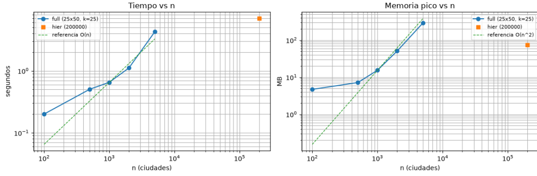
Figura 4: Tiempo y memoria frente a n (log-log) con referencias O(n) y O(n^2) , más el punto jerárquico de 200000.
