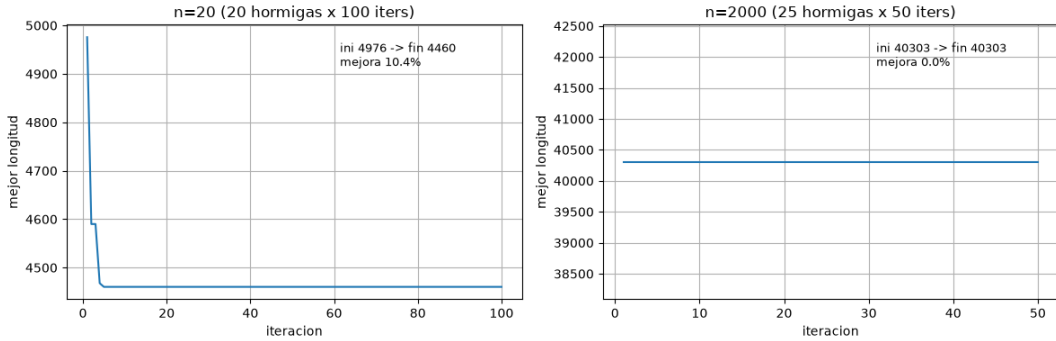
Figura 3: Mejor longitud global por iteración, n=20 y n=2000 .
