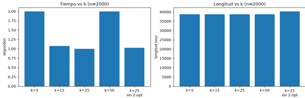
Figura 5: Tiempo y longitud según k ( n=2000 ), con variante sin 2-opt.
