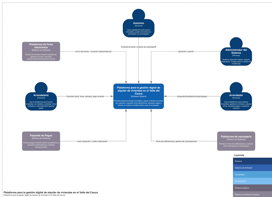
Figura 4.1: Vista de contexto C4 de la plataforma de gestión de arriendos
