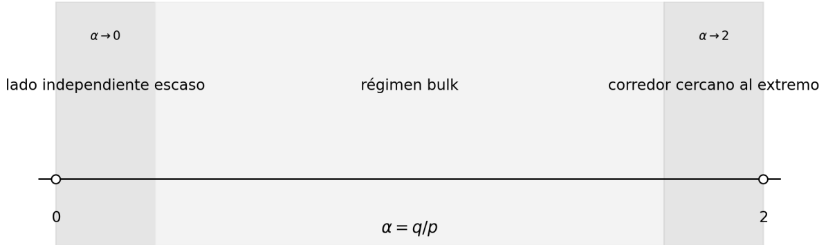
Figura 2: Mapa esquemático de los tres regímenes de la demostración sobre el eje de parámetros \alpha = q/p : el régimen escaso cerca de 0, el bulk alejado de ambos extremos y el corredor cercano al extremo cerca de 2.
