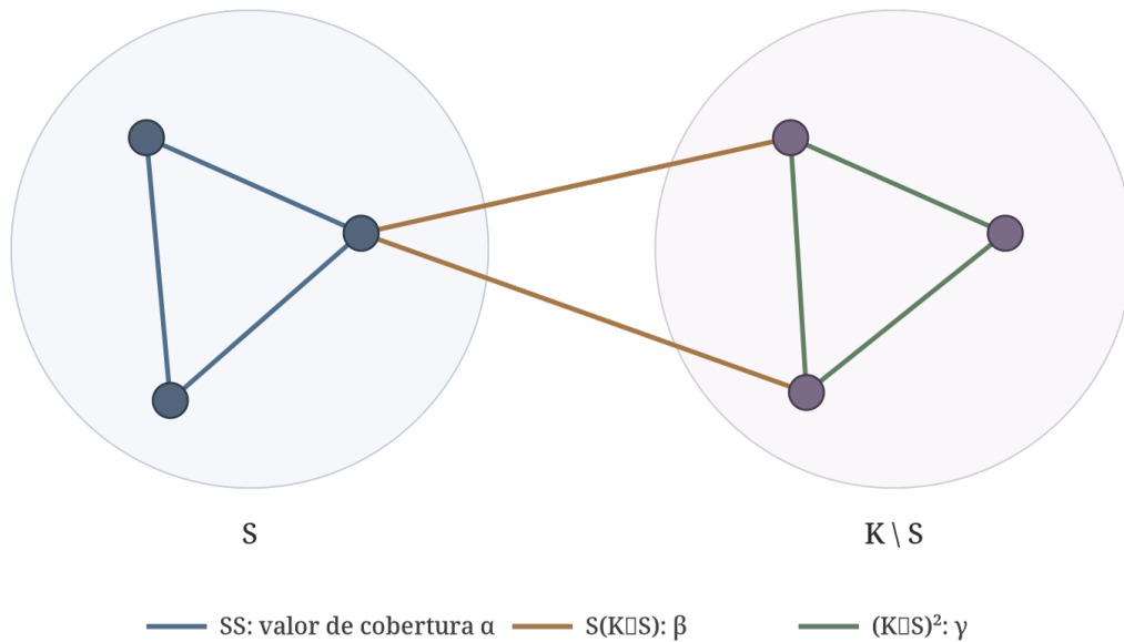
Figura 2: Las tres órbitas de aristas de un perfil puro.
