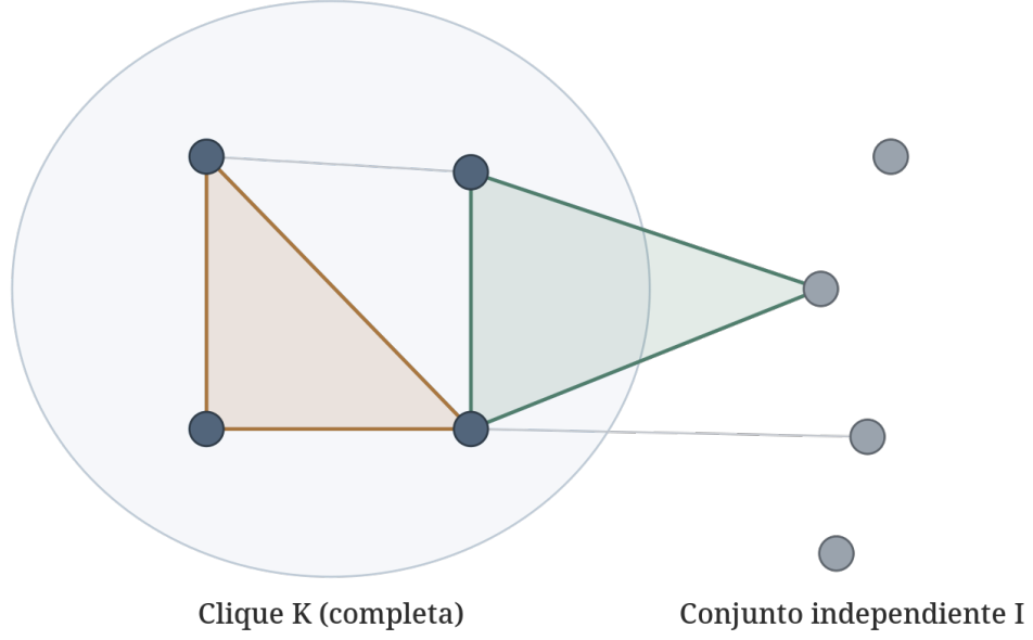
Figura 1: El empaquetamiento fraccional en dos fases.
