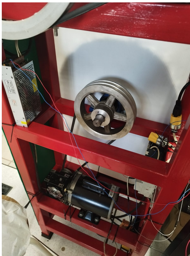
Imagen 64: Sistema de transmisión instalado
