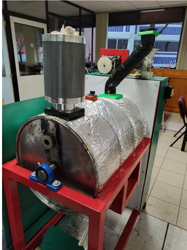
Imagen 66: Muestra del sistema de compostaje completo
