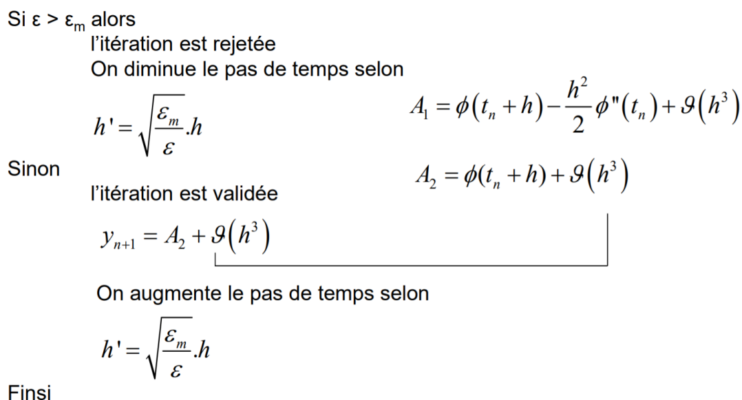
FIGURE 4 – Algorithme de la méthode RK12
