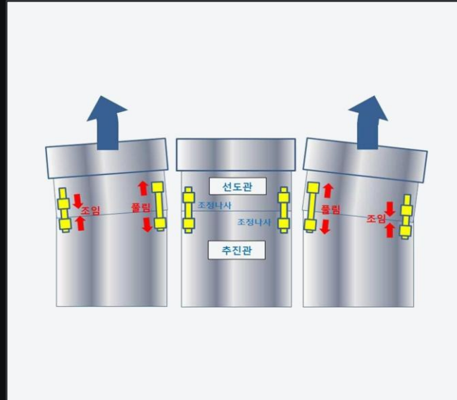
선도관 조정 원리 — 조임 · 풀림
