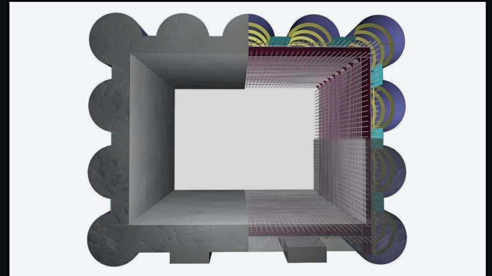
T.S.M 구조 개념도 — 강관 다발 내부 RC 박스 형성
