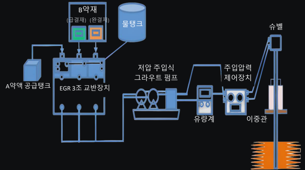
EGR 주입 계통도 — 교반·펌프·유량 제어·이중관
