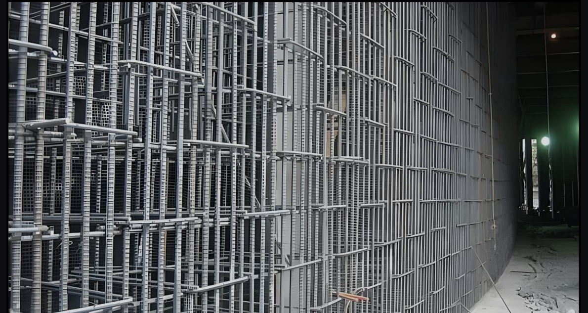
벽체 배근 상세
