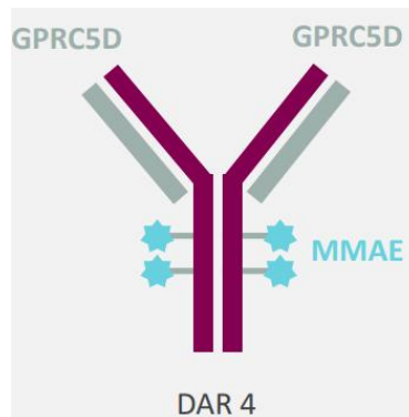
图4: LM-305/AZD0305 结构示意图
