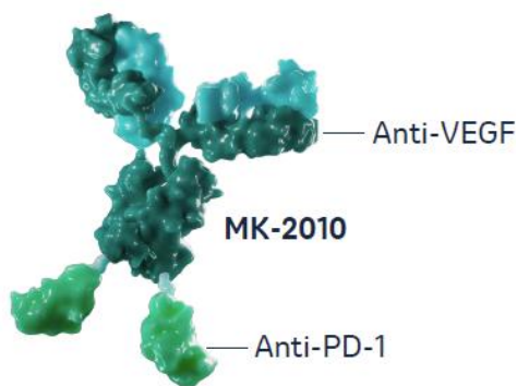
图3: LM-299/MK-2010 结构示意图
