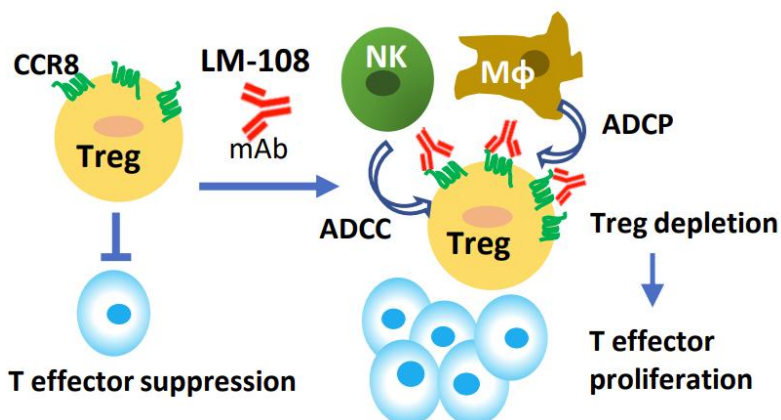
图5: LM-108 作用机制
