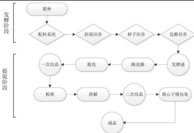
图12：硫氰酸红霉素的生产工艺流程
