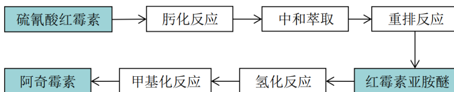
图9：公司生产阿奇霉素原料药的生产工艺流程
