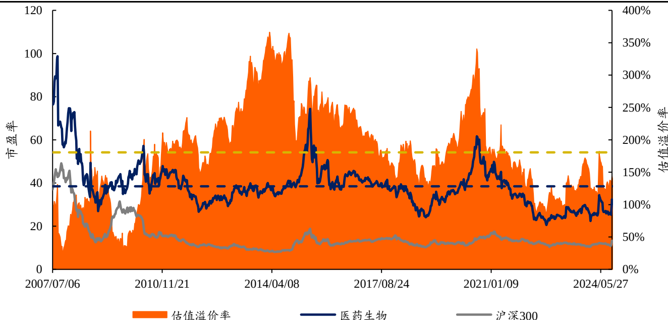
图7: 2007 年 7 月至今 (2025 年 5 月 16 日) 期间医药板块绝对估值水平变化
