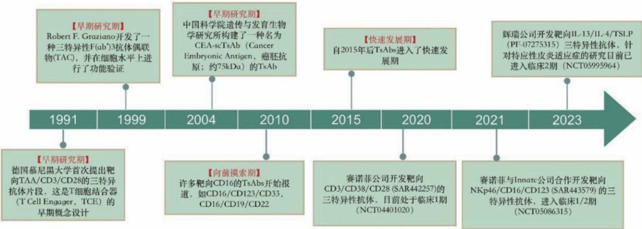
图1：三特异性抗体的发展趋势
