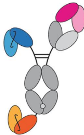
图4: JNJ-8543 抗体结构图
