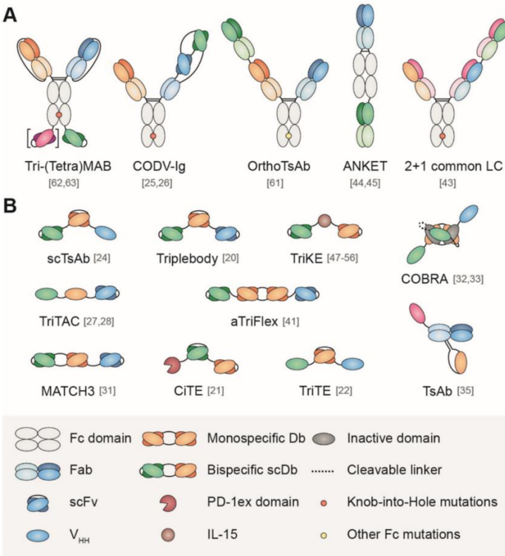
图2：包含（A）或不包含（B）Fc 结构域的多特异性抗体形式示意图
