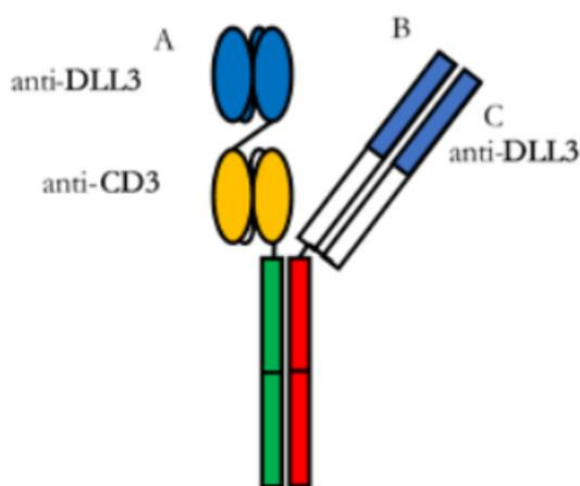
图3: ZG006 抗体结构图
