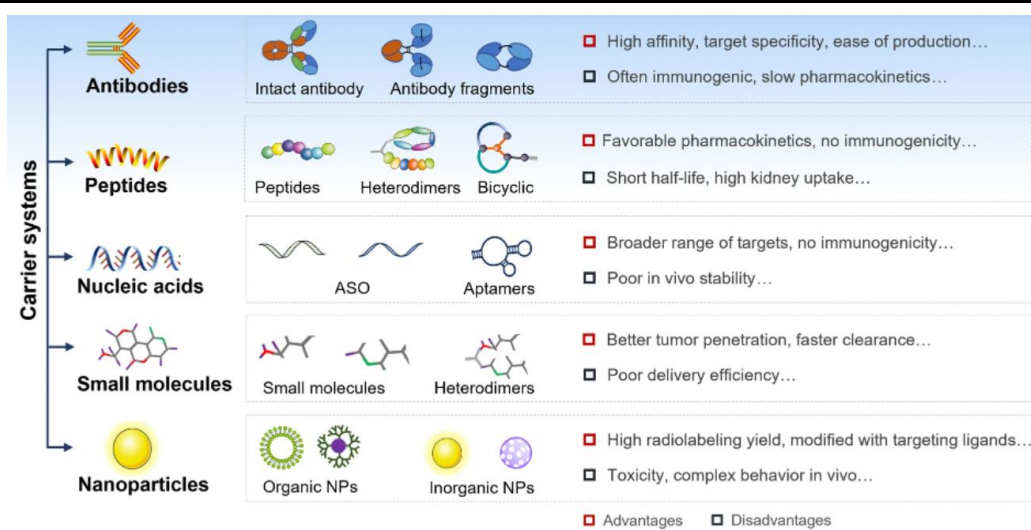
图1: RDC 的配体可选择性较多
