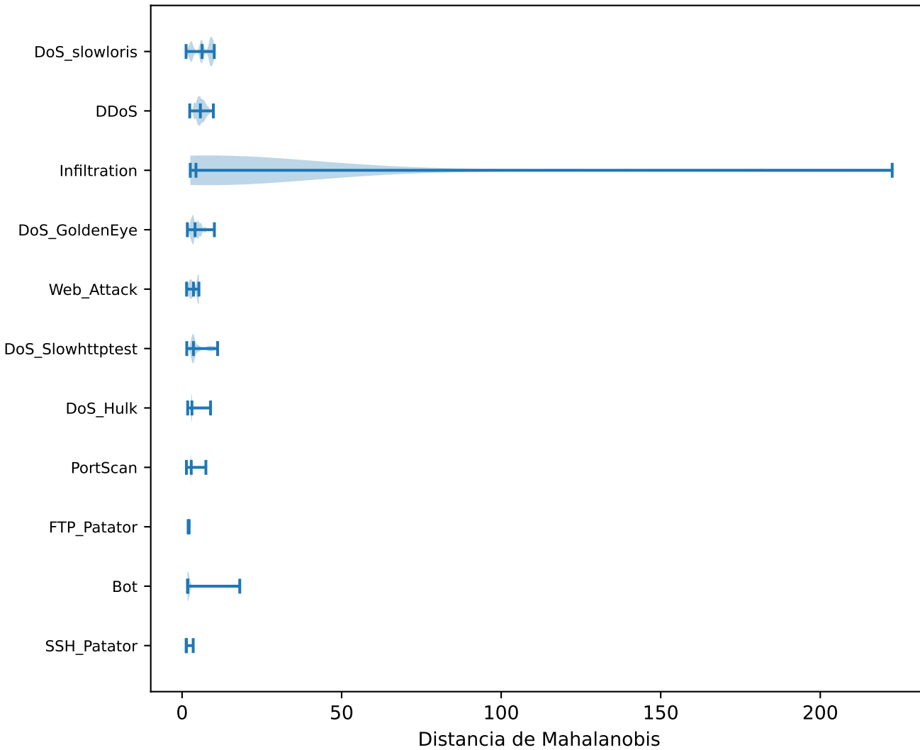
Distribución completa, seed=42
