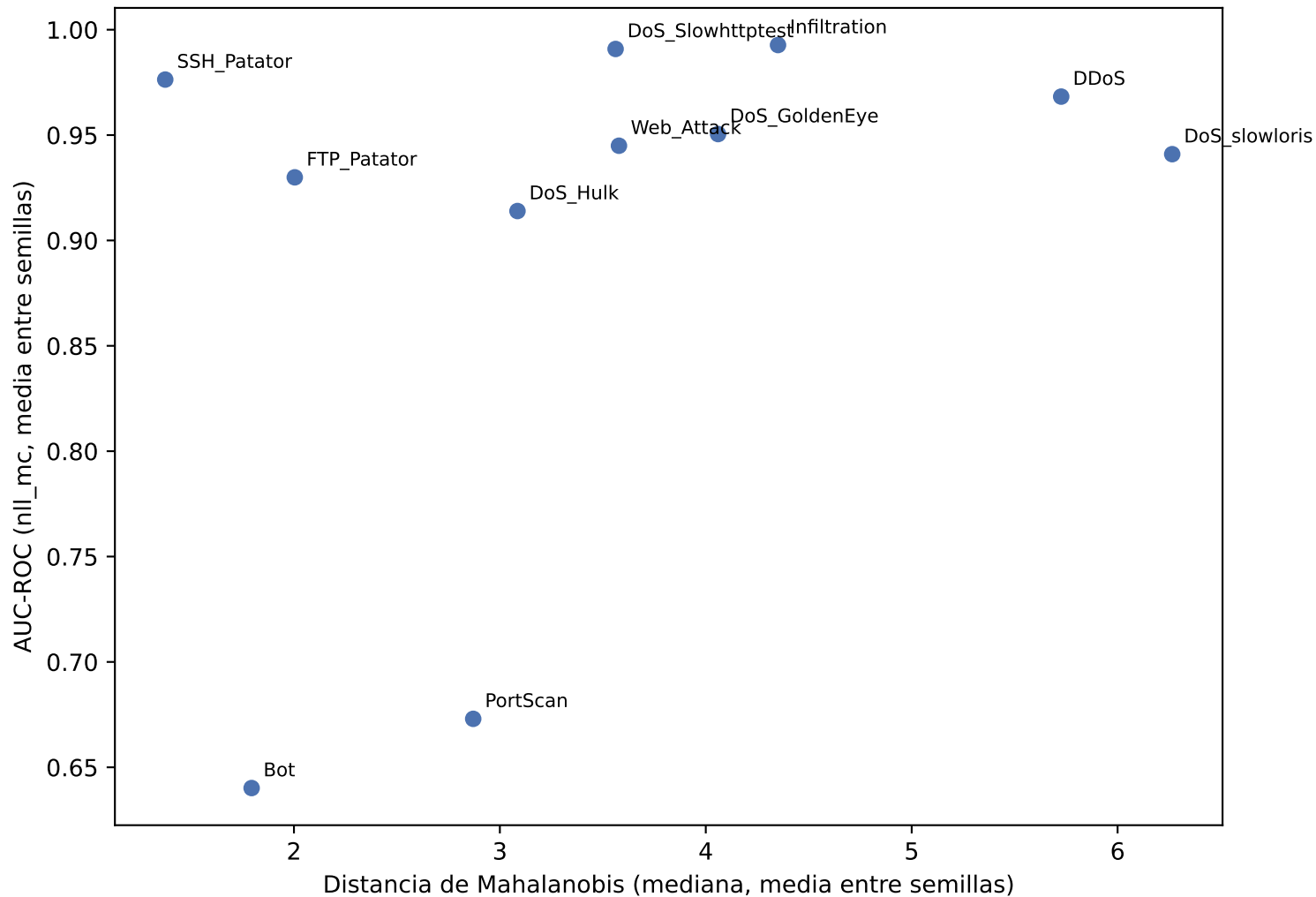
Geometría vs. detectabilidad, barras = DE entre semillas \rho combinado=0.382 IC95=[nan,nan]
