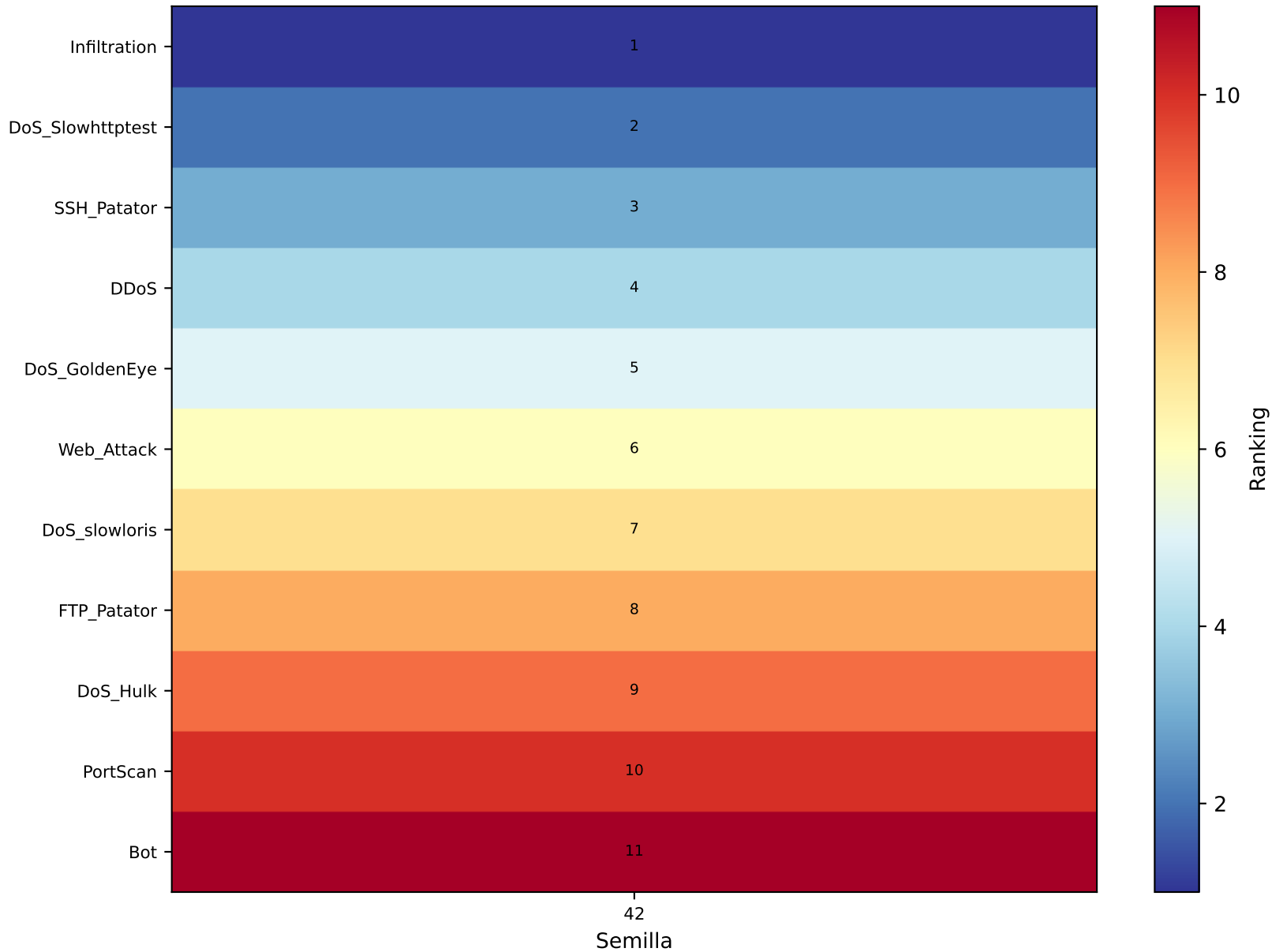
Ranking de detectabilidad (AUC-ROC nll_mc) por familia y semilla (1=más detectable)
